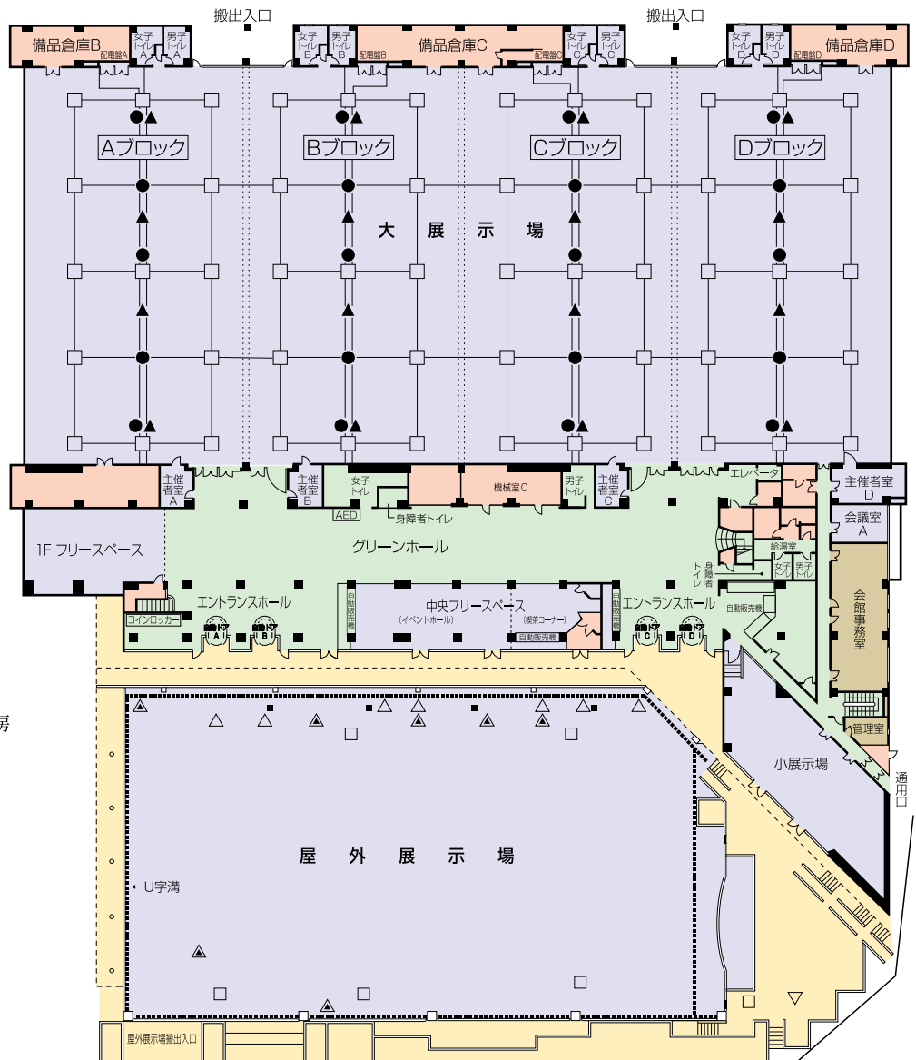
【1階平面図】
