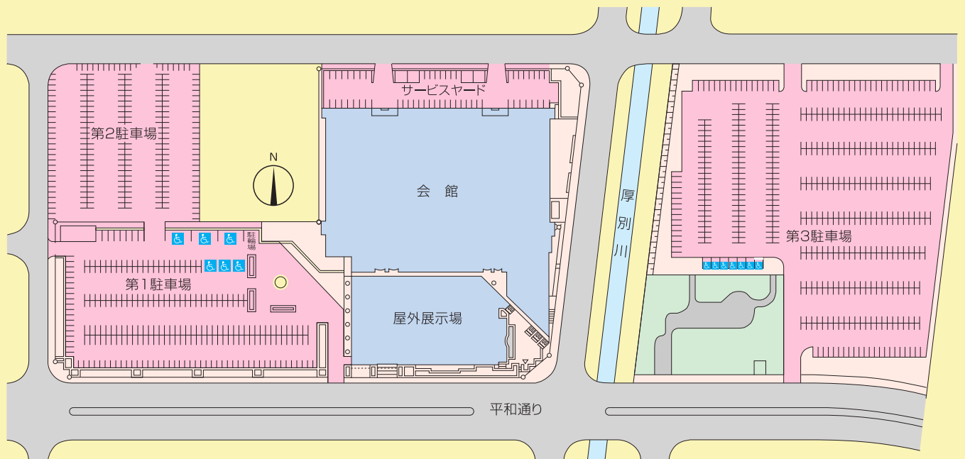
【建物配置図】
